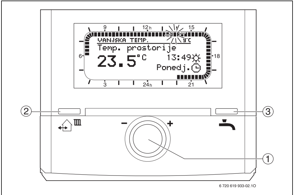
Sl. 2 Elementi rukovanja kod zatvorenog preklopnog poklopcia
