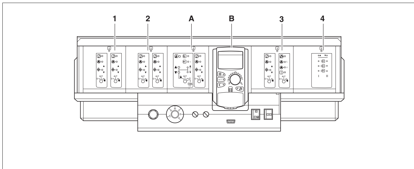
Sl. 5 Opremljenost modula
