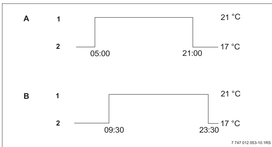
Sl. 20 Novi program grijanja
