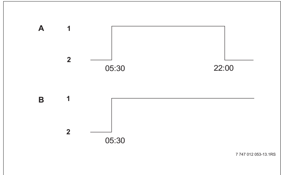
Sl. 17 Brisanje uklopne točke
