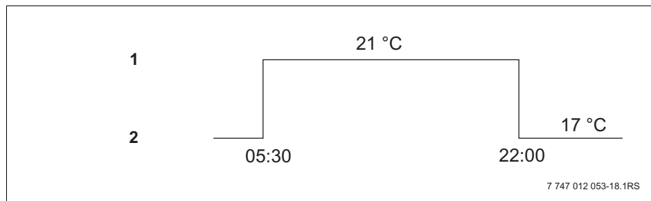
Sl. 9 Promjena sa dnevnog i noćnog pogona u fiksno utvrđena vremena na satu (primjer)
