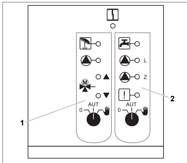
Sl. 22 Funkcijski modul FM441
