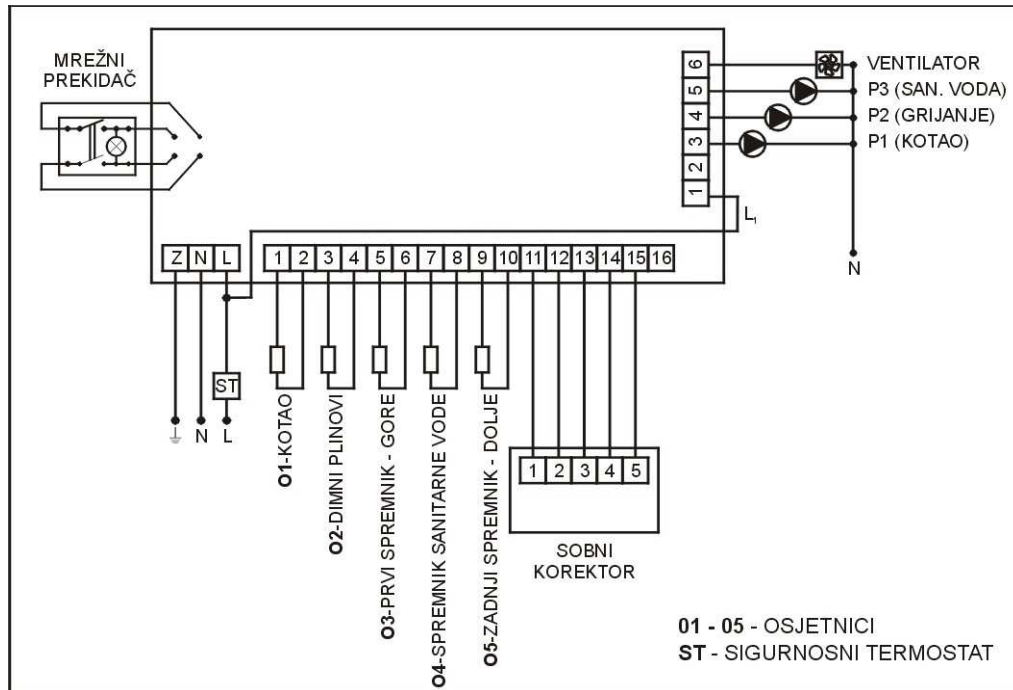
Slika 2. El. shema spajanja regulatora
